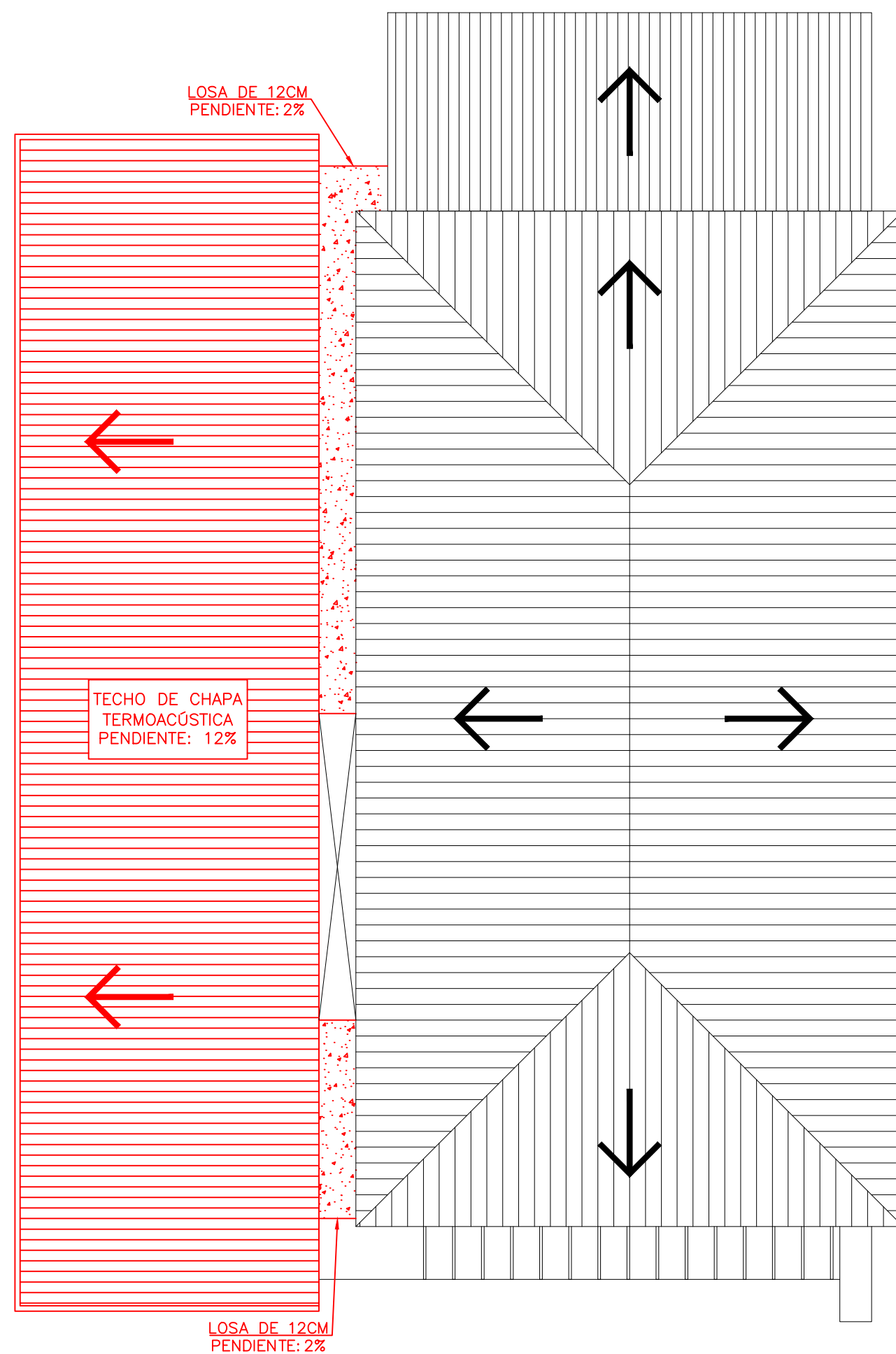
PLANTA DE TECHO ESC 1/100
