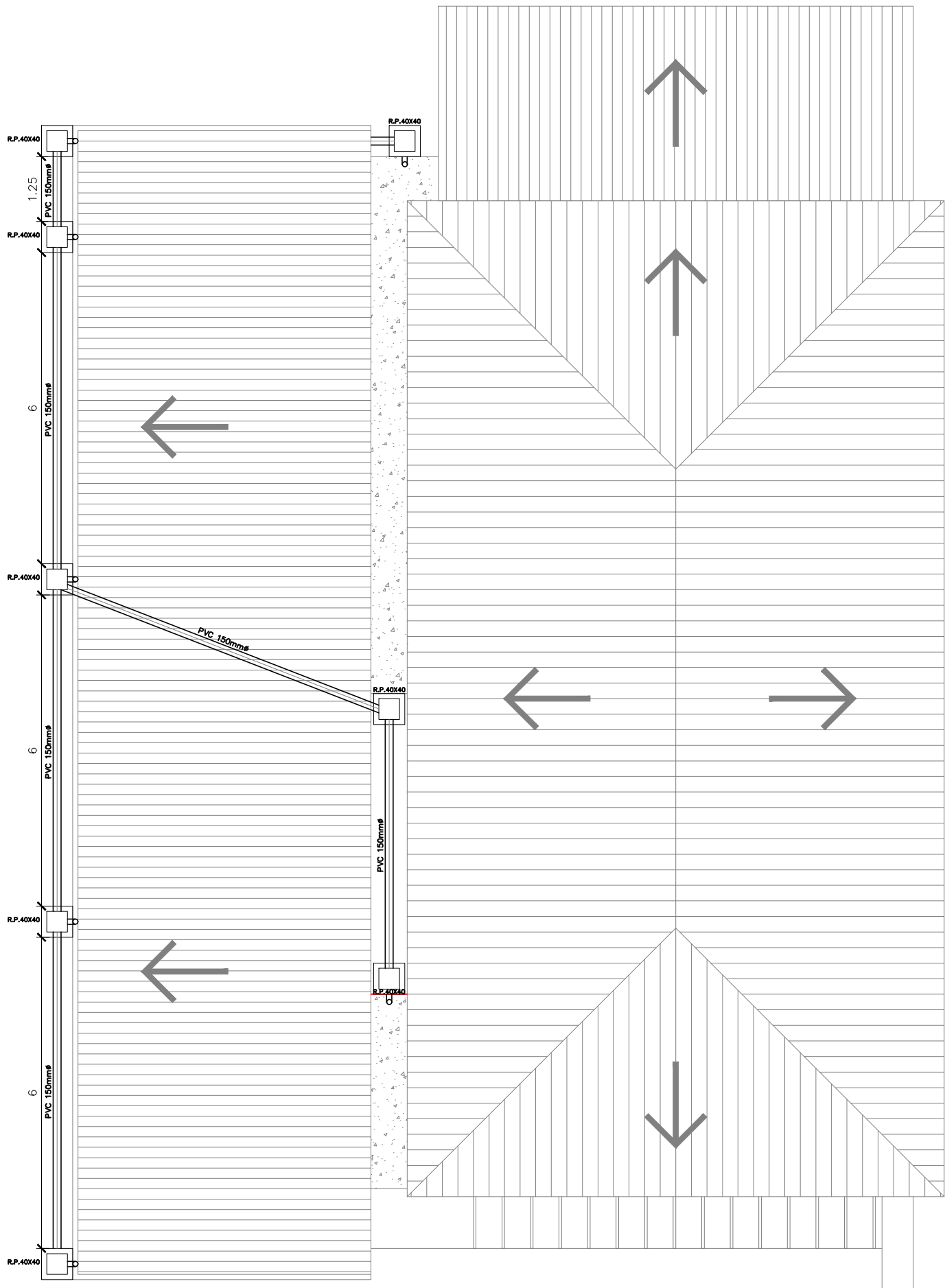
PLANTA DE DESAGÜE PLUVIAL ESC 1/100
