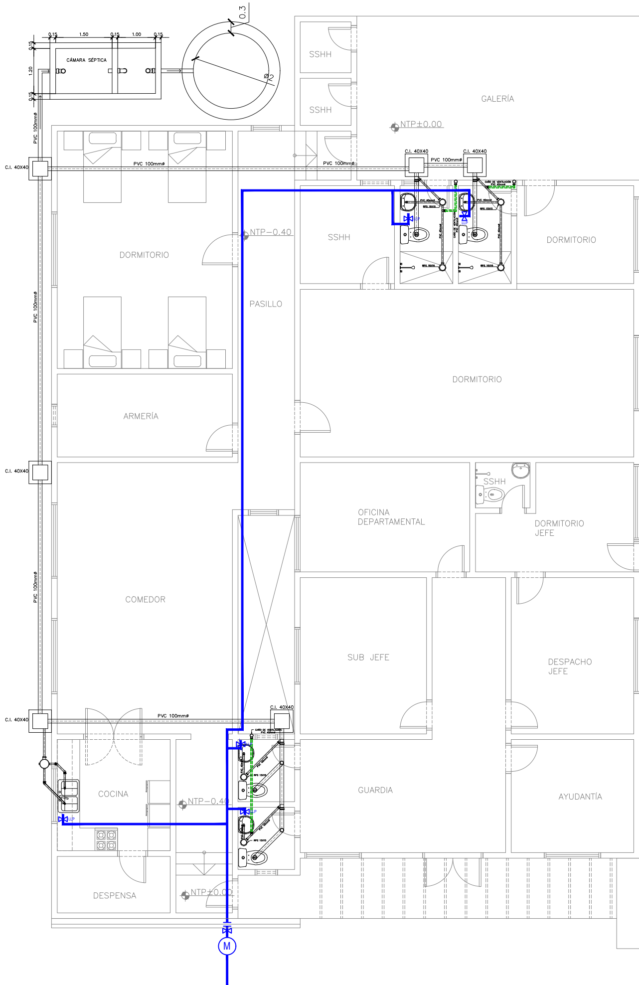
PLANTA HIDROSANITARIA ESC 1/100
