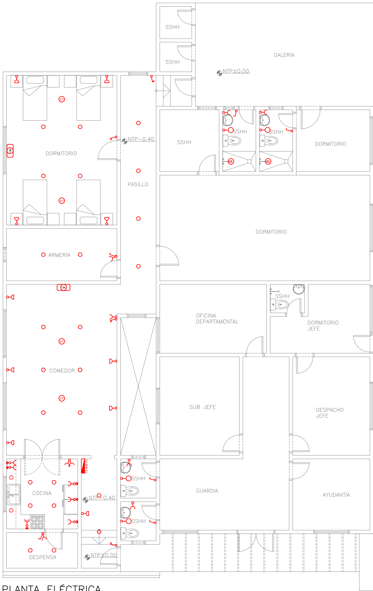
PLANTA ELÉCTRICA ESC 1/100
