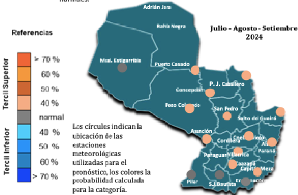
Figura 5. Pronóstico de Temperatura media trimestre IAS 2024.
