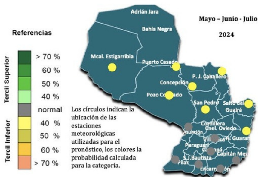
Figura 2. Pronóstico de Precipitación trimestre MJJ 2024
