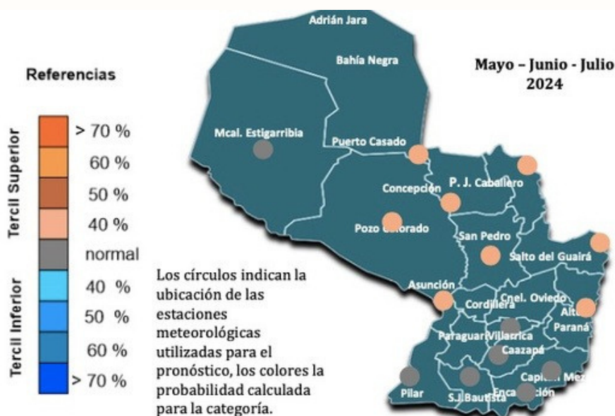
Figura 3. Pronóstico de Temperatura media trimestre MJJ 2024
