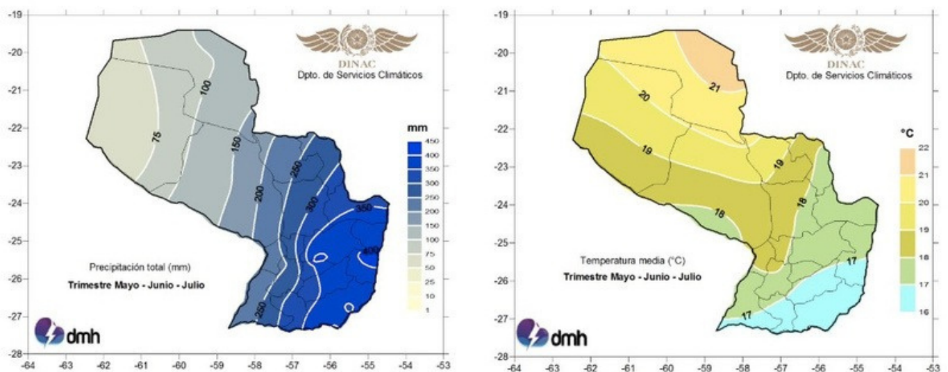
Figura 1. Precipitación total y temperatura trimestre MJJ 2024
