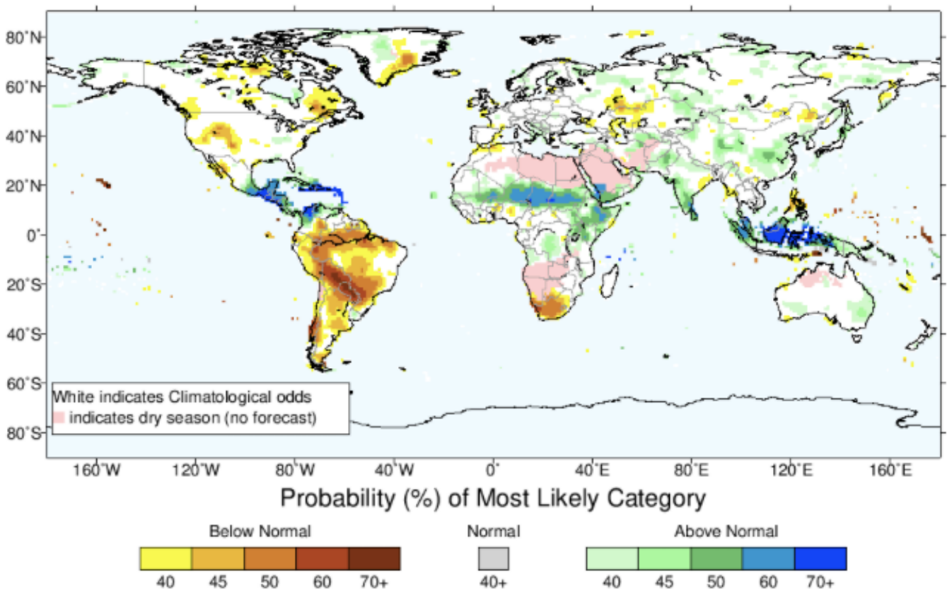
Figura 4. Pronóstico de probabilidad de precipitación multimodelo del IRI para Junio-julio-agosto de 2024, emitido en mayo de 2024. Fuente: International Research Institute for Climate and Society
