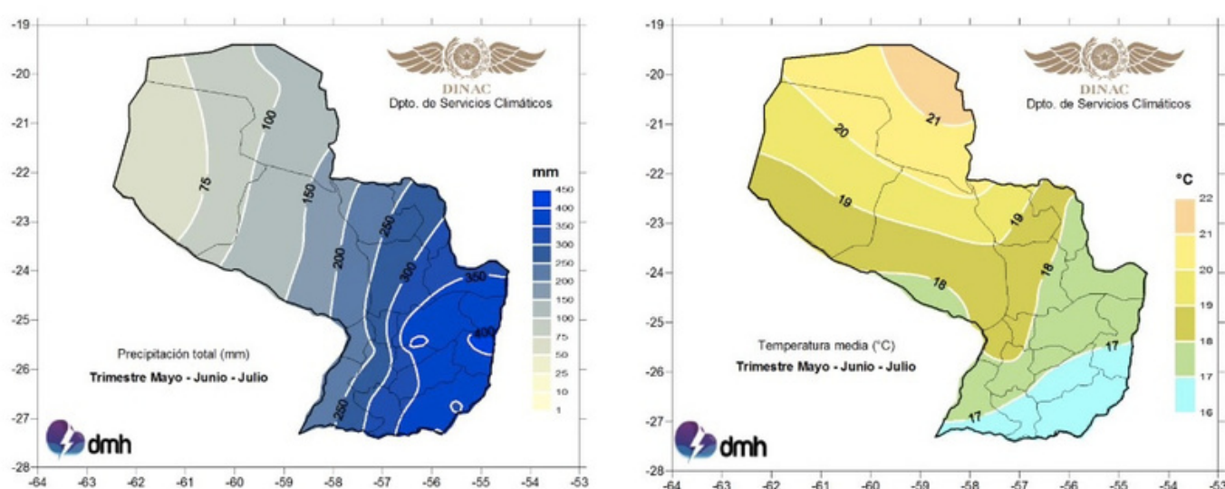
Figura 3. Precipitación total y temperatura trimestre MJJ 2024
