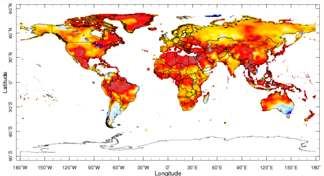
Figura 5. Pronóstico de temperatura estacional flexible emitido en Mayo de 2024.
