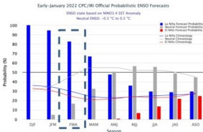
Figura 3. Probabilidad de fases del ENSO para la región de El Niño 3.4 actualizado al 13 de enero de 2022. Fuente: IRI (Instituto Internacional de Investigación para el Clima y la Sociedad)
