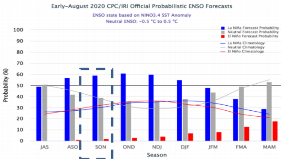
Figura 2. Probabilidad de fases del ENSO para la región de El Niño 3.4 actualizado al 13 de agosto de 2020. Fuente: IRI (Instituto Internacional de Investigación para el Clima y La Sociedad).
