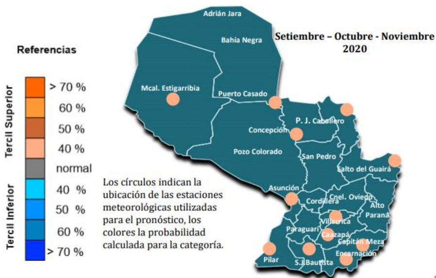
Figura 5. Pronóstico de Temperatura media trimestre SON 2020.
