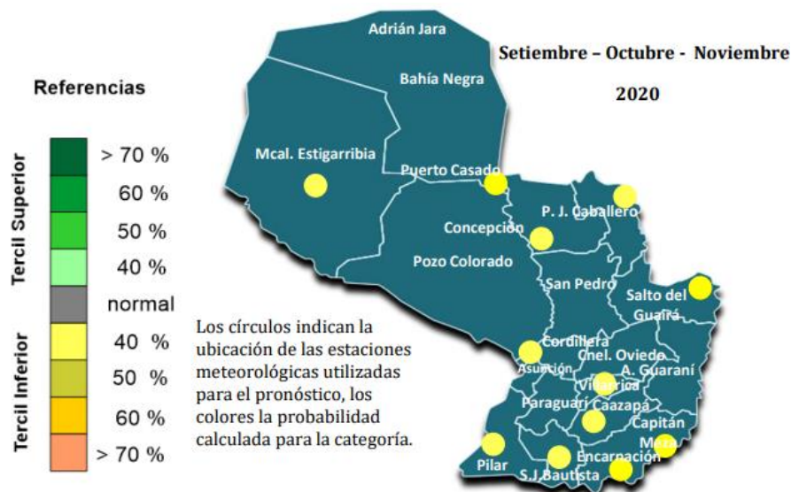
Figura 4. Pronóstico de Precipitación trimestre SON 2020.
